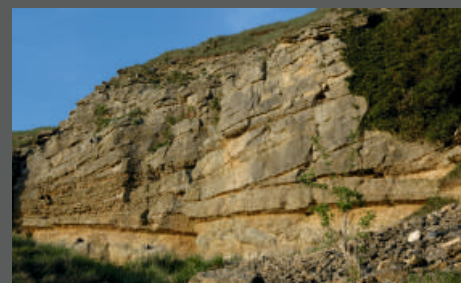
Oolite Deposystems
